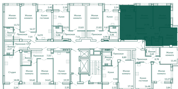
План этажа
